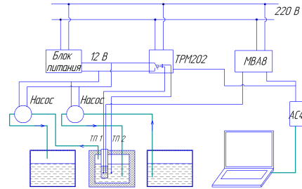
Электрическая схема лабораторного стенда для исследования процессов кристаллизации растворов
